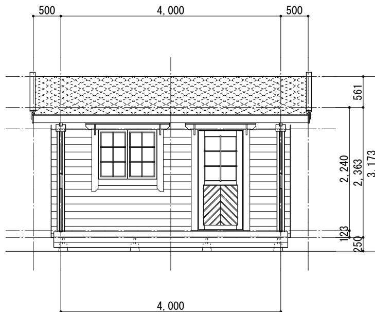
立面图 S=1/50
