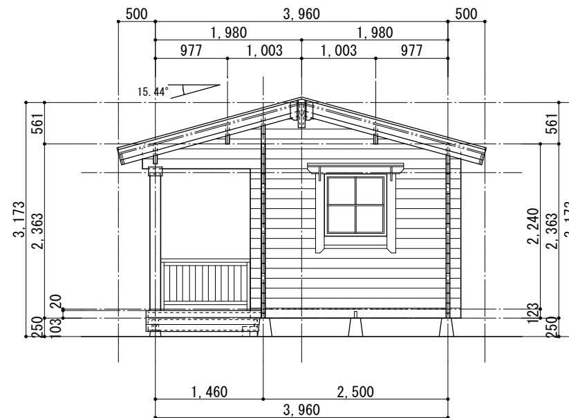
立面图 S=1/50
