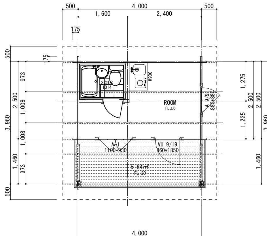
平面図 S=1/50
